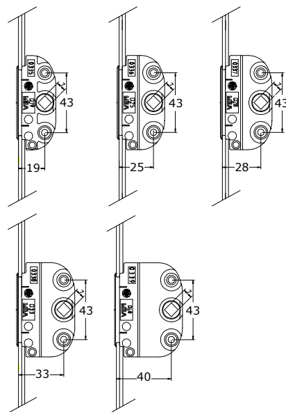
DORN / BACKSET
