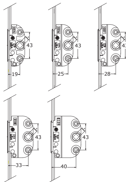
DORN / BACKSET
