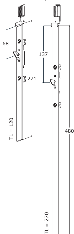
FORLÆNGERSTK. BUND EXTENSION, BOTTOM
