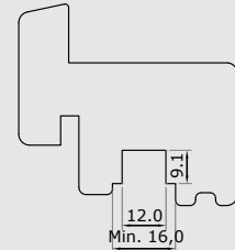
EKSEMPEL PÅ TRÆRAMME MED EURONOT. EXAMPLE OF TIM- BER FRAME WITH EURO GROOVE
