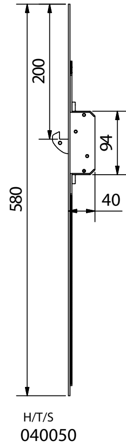
Topforlængere: Hoved-, terrasse- og halvdøre
