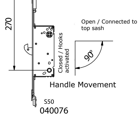
Stable Door Bottom
