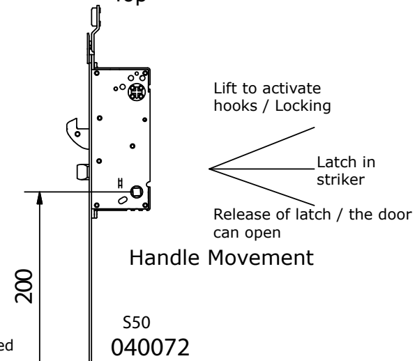
Stable Door Top
